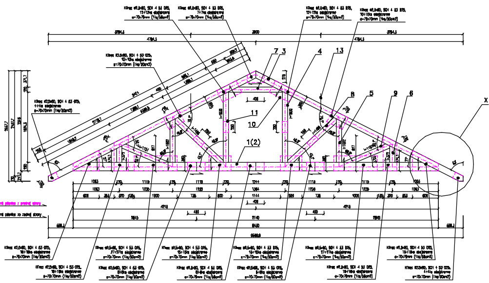
Přehradový nosník č. 2 M 126
